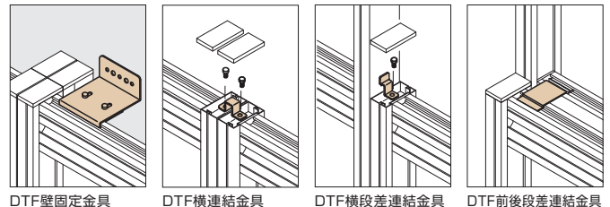
DTF壁固定金具
