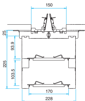
両面配線ダクト内 詳細
