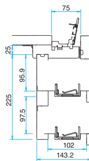
片面配線ダクト内 詳細
