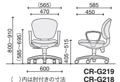
( ) 内は肘付きの寸法 CR-G219 CR-G218
